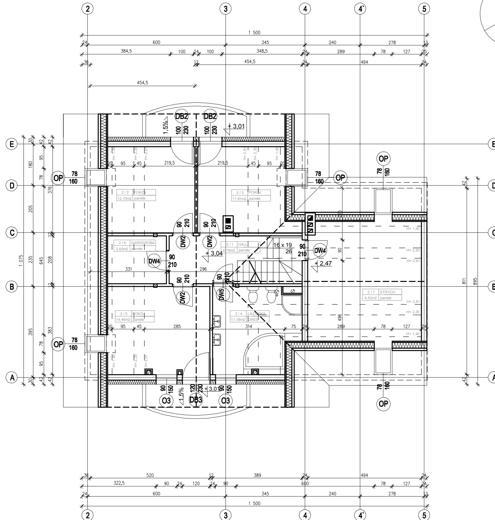
RZUT PODDASZA SKALA 1:100
